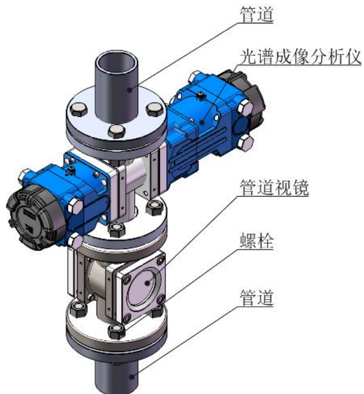
图 5 安装方式
