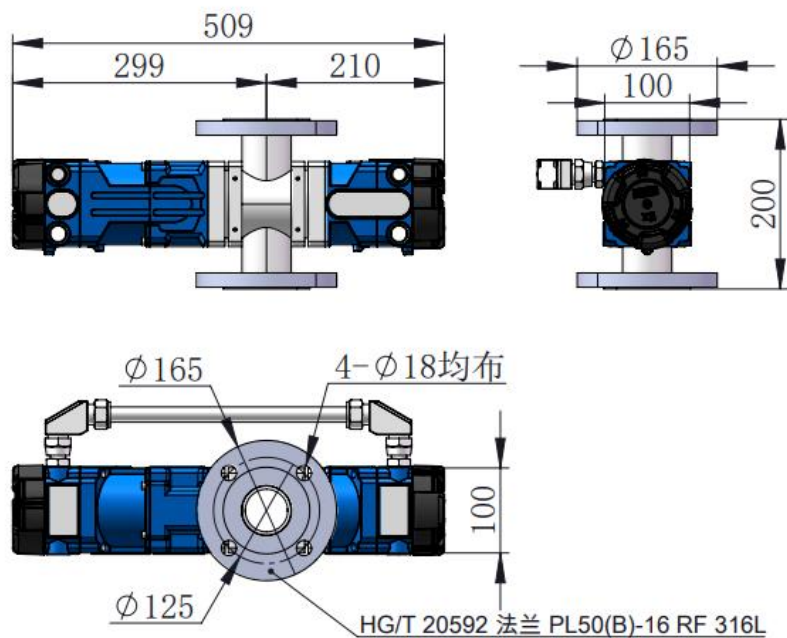
图 3 HST01 系列尺寸图
