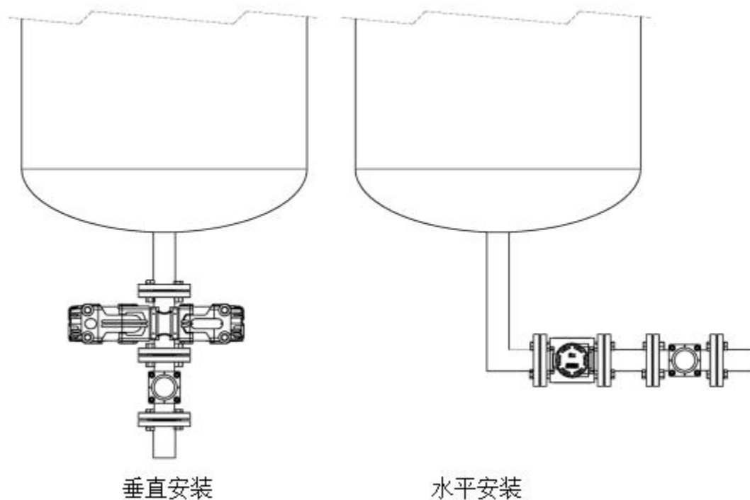
图 6 安装位置
