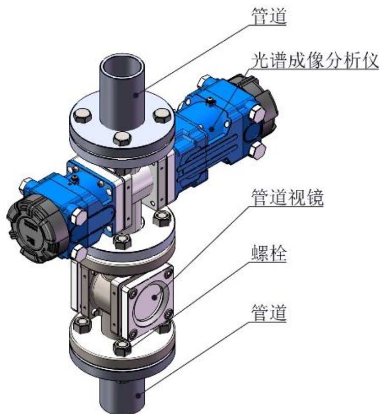
图 5 安装方式
