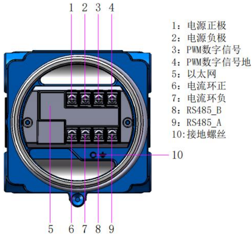
图 7 防爆视觉检测仪接线端子定义图
