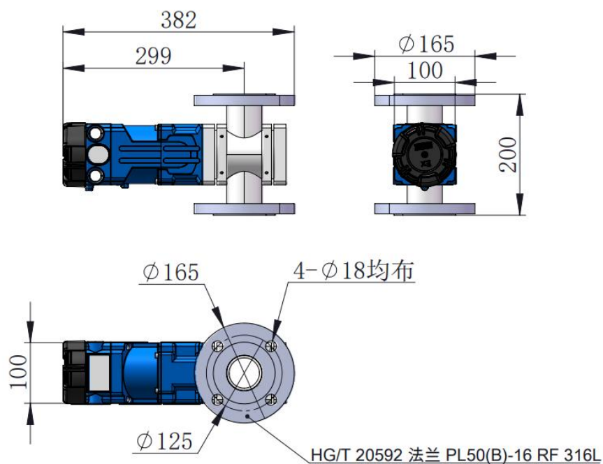
图 4 HSF02 系列尺寸图
